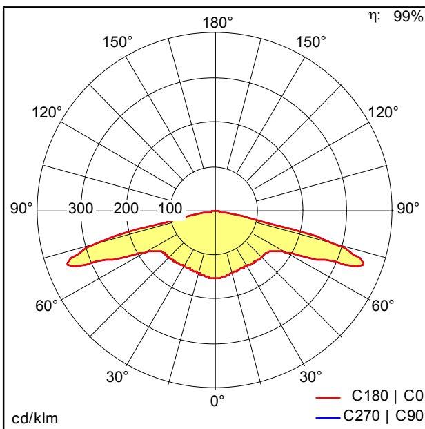
TE_IRIS_ANTIPANIC_SELFTEST_E3_LiFePO4.ltd
